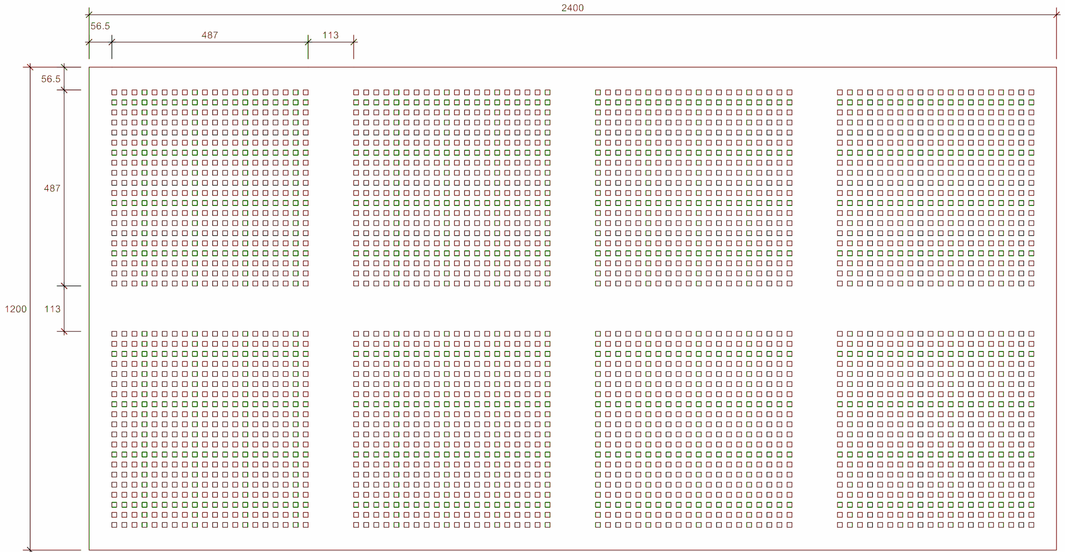
Gyptone Big Quattro 41 Scale 1:2
